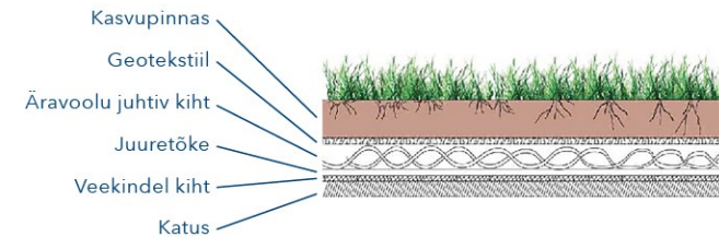
Joonis 5. Rohekatuse läbilõige.
