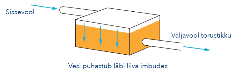
Joonis 19. Liivafiltri tööpõhimõte.
